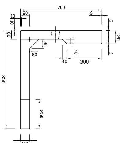
底版図
