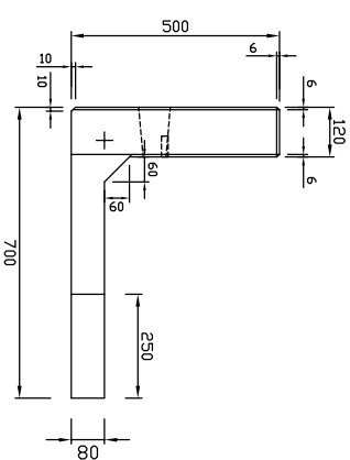
底版図
