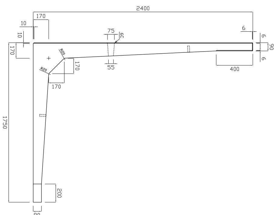
断面図
