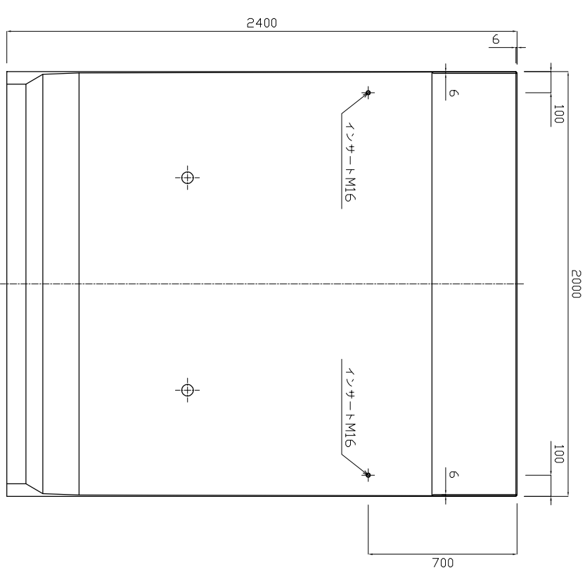
背面図
