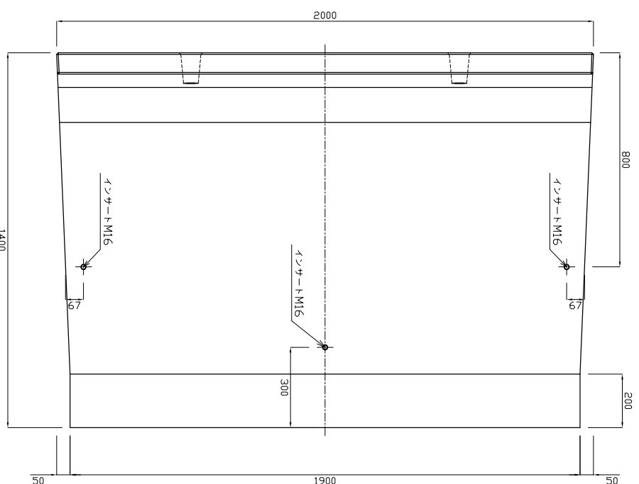
底版図
