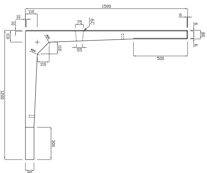
底版図
