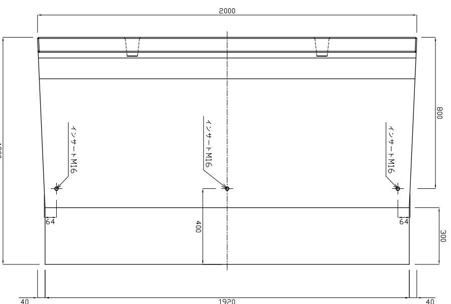
底版図
