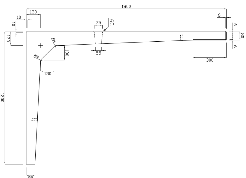
底版図
