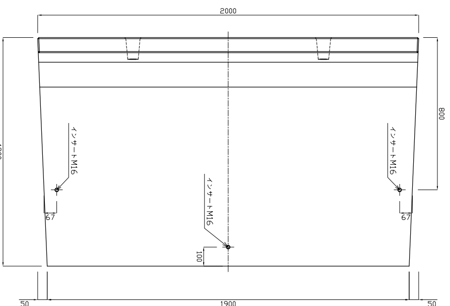
底版図
