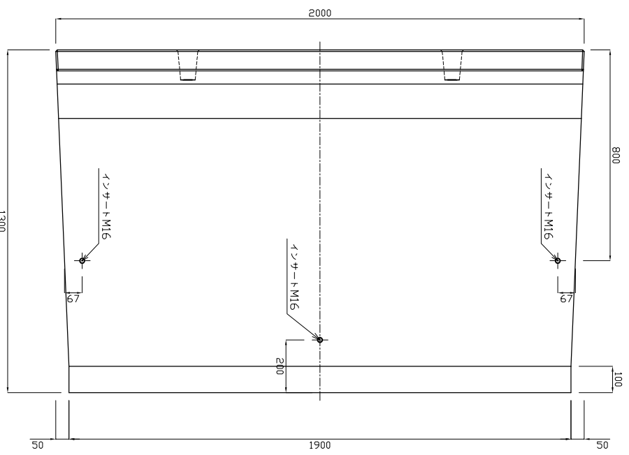
底版図
