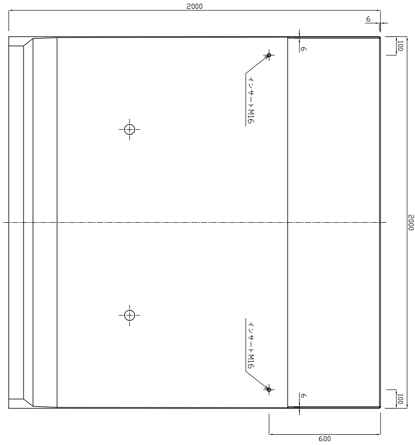
背面図
