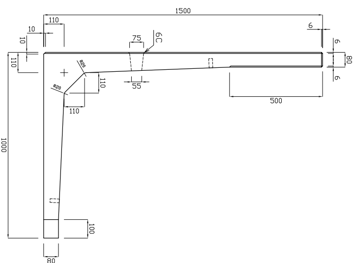
底版図
