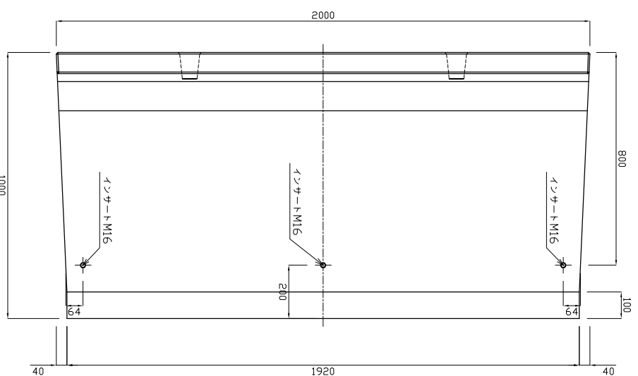
底版図
