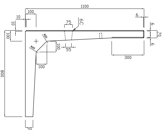
底版図
