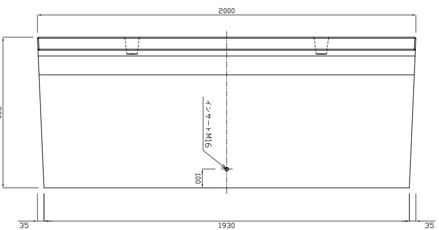
底版図
