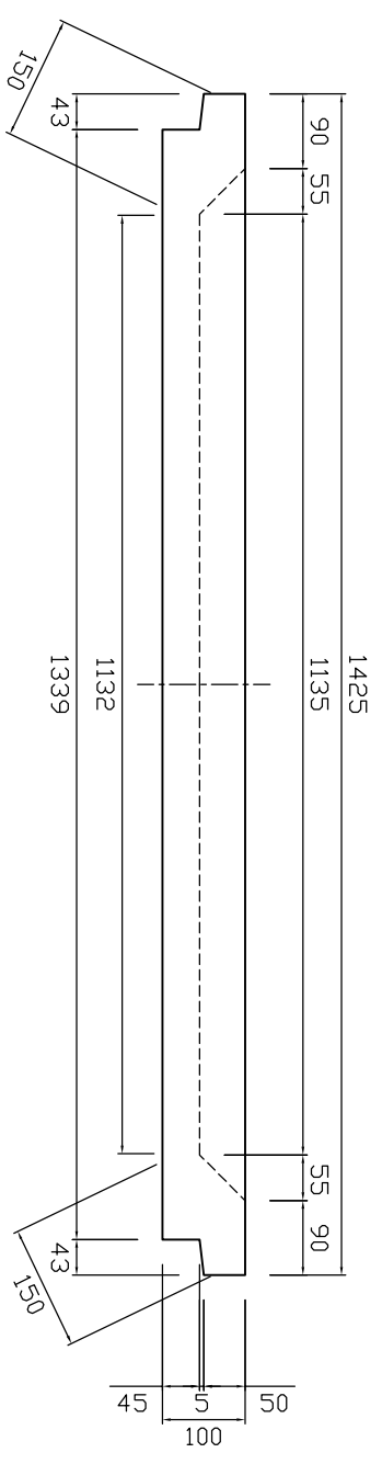
Q-Q'断面図
